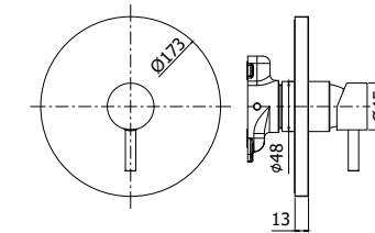
LIG BOX010CR Set esterno miscelatore incasso doccia senza deviatore External set for concealed shower mixer without diverter
