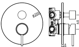
LIG 019CR Miscelatore incasso doccia (3 uscite) con cartuccia deviatore Concealed shower mixer (3 outlets) with diverter cartridge
