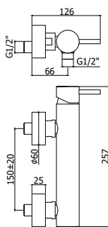
LIG 168-168DCR Miscelatore doccia esterno attacco 1/2" con/senza set doccia Shower mixer 1/2" connection with/without shower set
