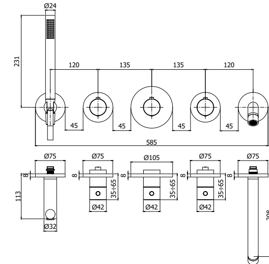
MDE 001 Set esterno per miscelatore termostatico incasso doccia/vasca (2 funzioni) - Installazione solo orizzontale External set for concealed thermostatic shower/bath mixer (2 functions) - Horizontal installation only
