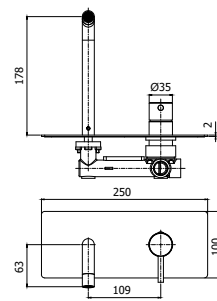
LIG 105-104-106CR Miscelatore incasso con bocca erogazione a muro 178 mm / 123 mm / 248 mm Concealed wash basin mixer with wall spout 178 mm / 123 mm / 248 mm
