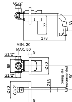
LIG 006-007CR70 Miscelatore incasso con bocca erogazione a muro 178 mm / 248 mm Concealed two-hole basin mixer with wall spout 178 mm / 248 mm
