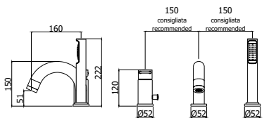
JK 040L-041LCR Miscelatore bordo vasca con doccia estraibile, con/senza bocca erogazione Deck mounted bath mixer with pull out hand-shower, with/without spout
