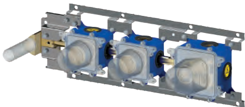
MDBOX 000 Set incasso per miscelatore termostatico doccia/vasca (2 funzioni) - Installazione solo orizzontale Concealed set for thermostatic shower/bath mixer (2 functions) - Horizontal installation only
