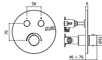
CPM 018CR Set esterno miscelatore incasso doccia (2 funzioni) con deviatore a pulsante On/Off External set for concealed shower mixer (2 functions) with push diverter On/Off
