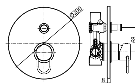
JK 015CR Miselatore incasso doccia (2 uscite) con deviatore a pulsante Concealed shower mixer (2 outlets) with push diverter
