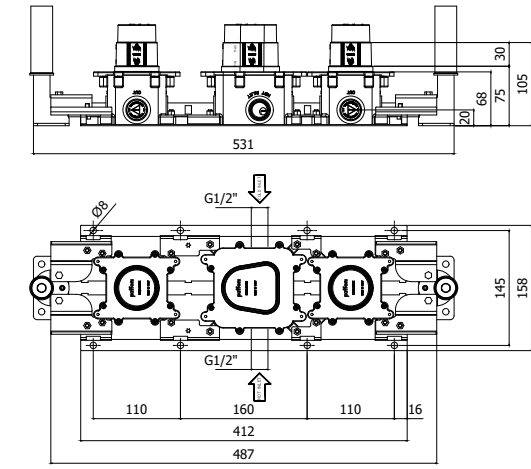
MDBOX 001 Set incasso per miscelatore termostatico doccia/vasca (2 funzioni) - Installazione solo orizzontale Concealed set for thermostatic shower/bath mixer (2 functions) - Horizontal installation only
