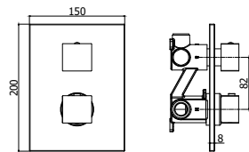
LEQ 518-519CR Miscelatore termostatico incasso doccia con deviatore 2 uscite/3 uscite Concealed thermostatic shower mixer with diverter 2 outlets/3 outlets
