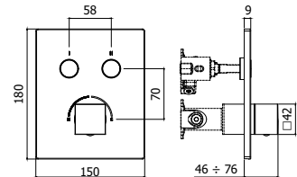
CPM 518CR Set esterno miscelatore incasso doccia (2 funzioni) con deviatore a pulsante On/Off External set for concealed shower mixer (2 functions) with push diverter On/Off
