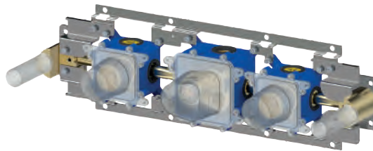
MDBOX 001 Set incasso per miscelatore termostatico doccia/vasca (2 funzioni) - Installazione solo orizzontale Concealed set for thermostatic shower/bath mixer (2 functions) - Horizontal installation only
