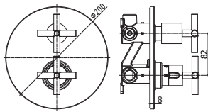
QTV 018CR Miscelatore termostatico incasso doccia con deviatore 2 uscite Concealed thermostatic shower mixer with diverter 2 outlets
