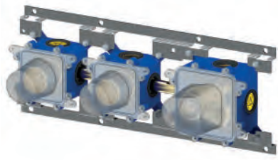
MDBOX 018 Set incasso per miscelatore termostatico doccia/vasca (2 funzioni) - Installazione orizzontale o verticale Concealed set for thermostatic shower/bath mixer (2 functions) - Horizontal or vertical installation
