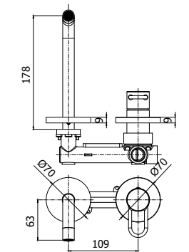
JK 105-104-106CR70 Miscelatore incasso con bocca erogazione a muro 178 mm / 123 mm / 248 mm Concealed wash basin mixer with wall spout 178 mm / 123 mm / 248 mm
