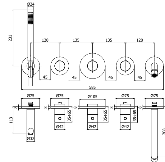
MDE 001 Set esterno per miscelatore termostatico incasso doccia/ vasca (2 funzioni) - Installazione solo orizzontale External set for concealed thermostatic shower/bath mixer (2 functions) - Horizontal installation only
