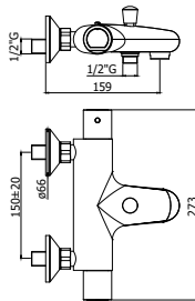
EQS 022-023CR Miscelatore termostatico vasca/doccia attacco 1/2" con senza set doccia Thermostatic bath/shower mixer 1/2" connection with without shower kit
