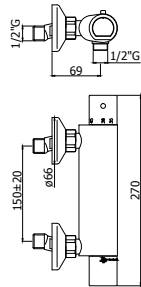
EQS 168-168DCR Miscelatore termostatico doccia attacco 1/2" con senza set doccia Thermostatic shower mixer 1/2" connection with without shower kit
