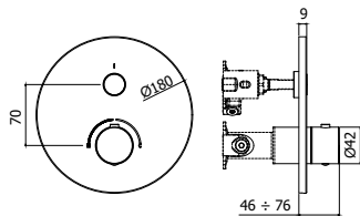
CPM 013CR Set esterno miscelatore incasso doccia (1 funzione) con deviatore a pulsante On/Off External set for concealed shower mixer (1 function) with push diverter On/Off
