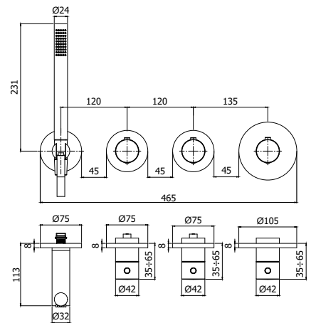
MDE 000 Set esterno per miscelatore termostatico incasso doccia/ vasca (2 funzioni) - Installazione solo orizzontale External set for concealed thermostatic shower/bath mixer (2 functions) - Horizontal installation only
