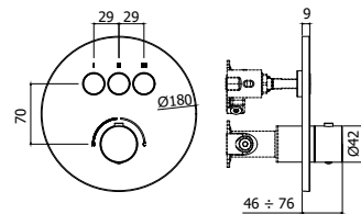
CPM 019CR Set esterno miscelatore incasso doccia (3 funzioni) con deviatore a pulsante On/Off External set for concealed shower mixer (3 functions) with push diverter On/Off
