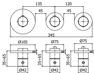
MDE 018CR Set esterno per miscelatore termostatico incasso doccia/ vasca (2 funzioni) - Installazione orizzontale o verticale External set for concealed thermostatic shower/bath mixer (2 functions) - Horizontal or vertical installation
